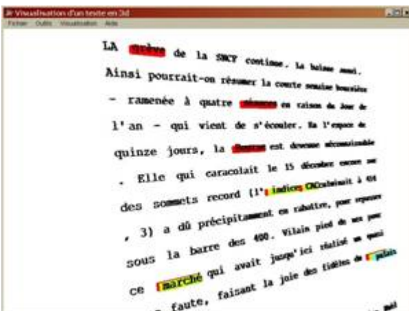
Figure 4 – 3D-LUCIAVizualizer : vue en trois dimensions des redondances de valeurs d'attributs.
