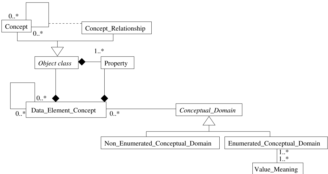
FIG. 2 – Diagramme de classes UML du niveau métadonnées conceptuelles de l'ISO11179-3
