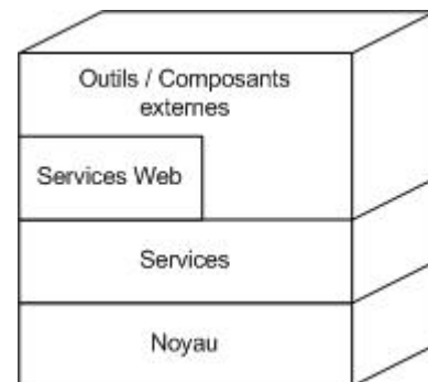
FIG. 6 – Niveaux d'abstraction de COW
