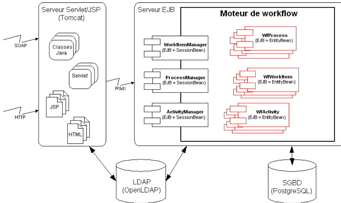
FIG. 5 – Architecture du moteur de workflows
