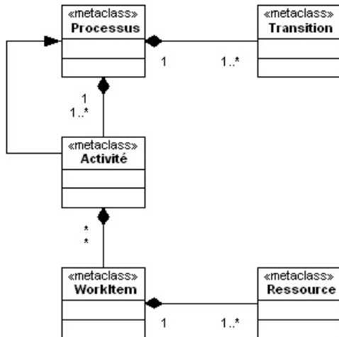
FIG. 3 – Méta-modèle de COW
