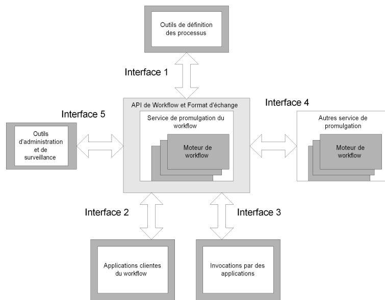
FIG. 1 – Modèle de référence des systèmes de workflow ([7])
