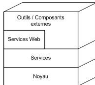
FIG. 6 – Niveaux d'abstraction de COW
