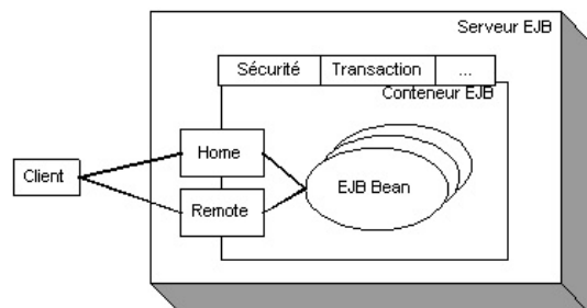
FIG. 4 – Représentation schématique d'un serveur EJB
