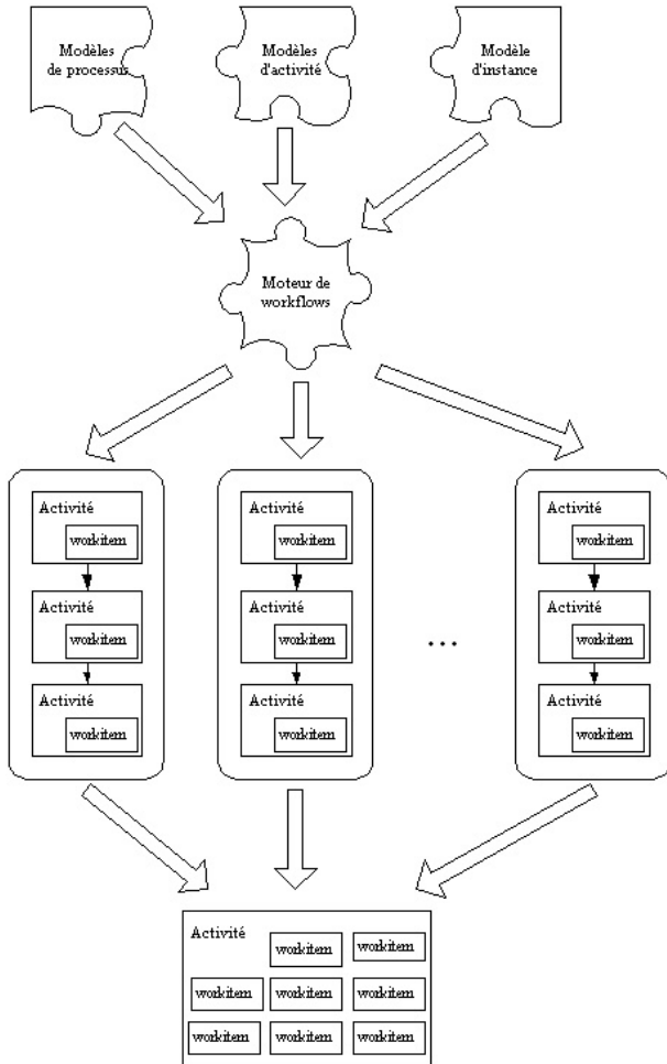
FIG. 9 – Instantiation des modèles
