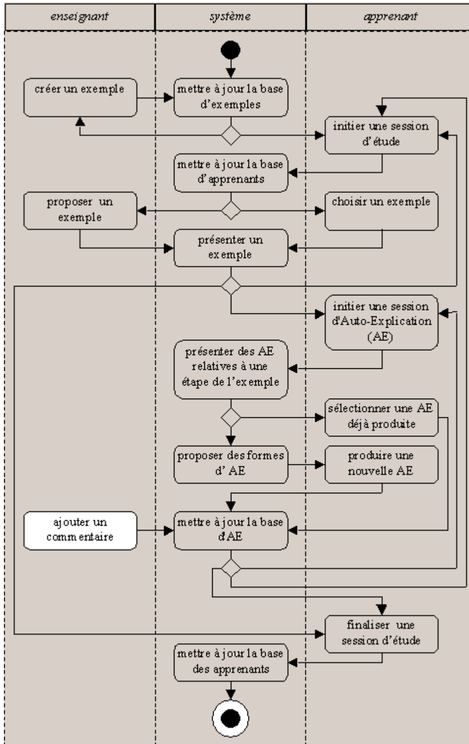
Figure 1. Diagramme d'activités.
